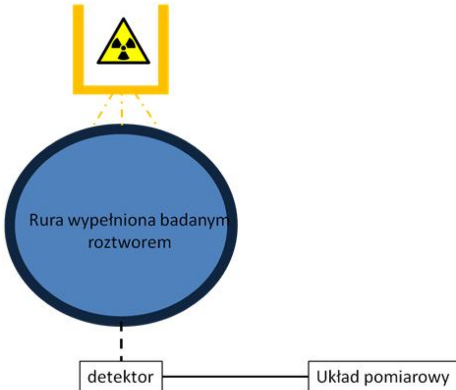
Rys. 5 Miernik gęstości
